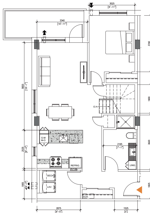
Rez-de chaussé
